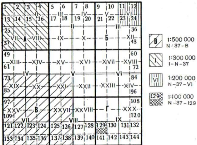
Рис. 43. Общая схема разграфки листа миллионной карты
