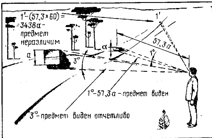
Рис. 14. Различимость предметов
