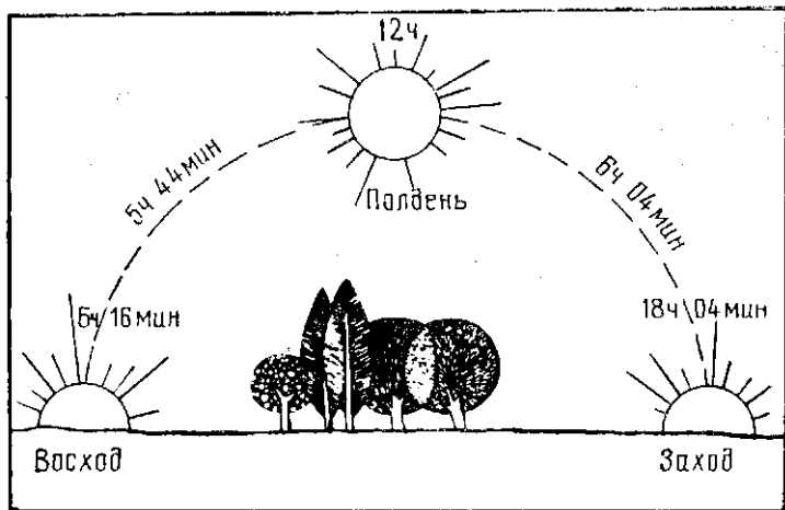
Рис. 48. Продолжительность дня и полдень по местному времени на широте 35^\circ (12 марта)
