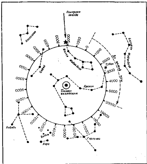
Рис. 50. Странствующий Северный полюс мира
