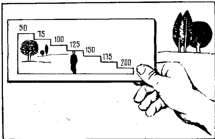
Рис. 27. Пластинка Лионде
