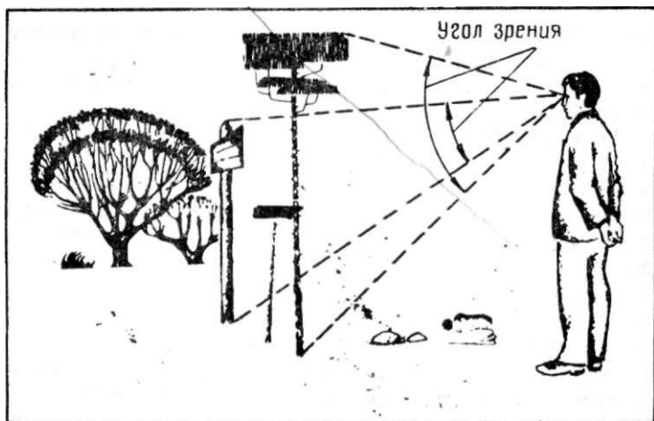
Рис. 13. Угол зрения
