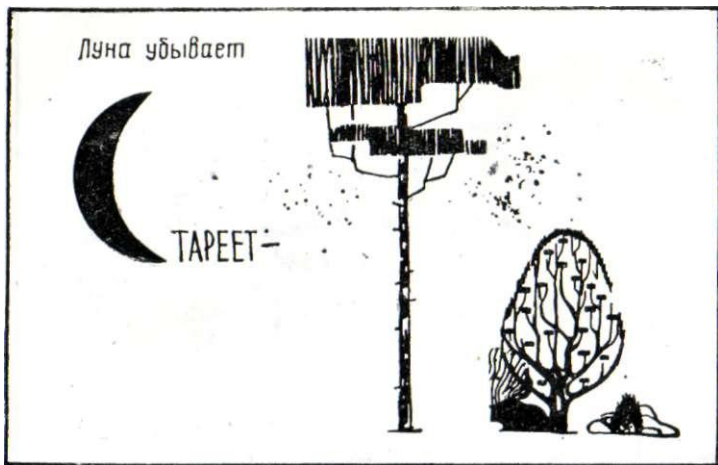
Рис. 60. Луна убывает
