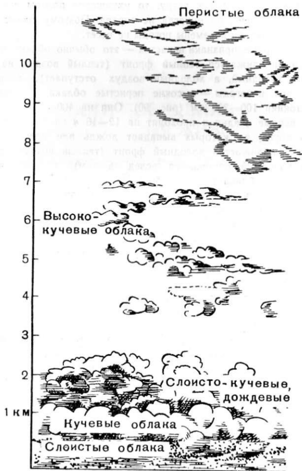
Рис. 90. Облака
